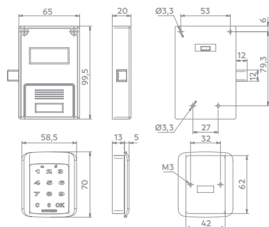
Fechadura Digital para Móveis 1701 Com Puxador
