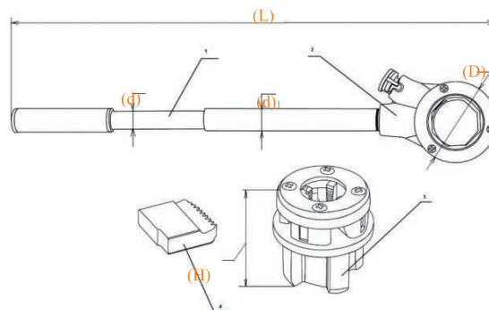
1-Cabo; 2-Corpo da base; 3-Mandril para cortadores; 4-Pestana de corte.
