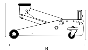
51133 : altura min.135 mm - max.465 mm 51135 : altura min.100mm - max.565 mm
