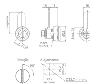
FECHO LINGUETA TRIÂNGULO LINGUETA COM DOBRA 7MM
