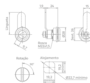
FECHO LINGUETA TRIÂNGULO LINGUETA COM DOBRA 2MM
