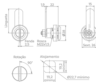
FECHO LINGUETA FENDA LINGUETA RETA
