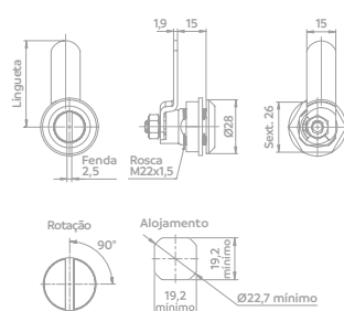
FECHO LINGUETA FENDA LINGUETA COM DOBRA 7MM
