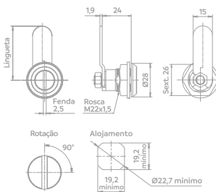
FECHO LINGUETA FENDA LINGUETA COM DOBRA 2MM
