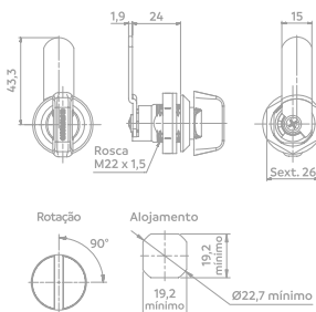
FECHO LINGUETA COM ACIONADOR LINGUETA COM DOBRA 2MM
