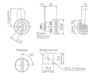
FECHO LINGUETA TRIÂNGULO LINGUETA RETA
